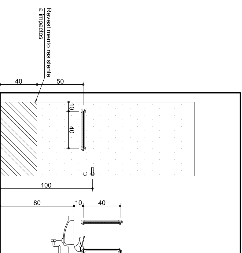
BANHEIRO PNE VISTA 3 escala 1/25
