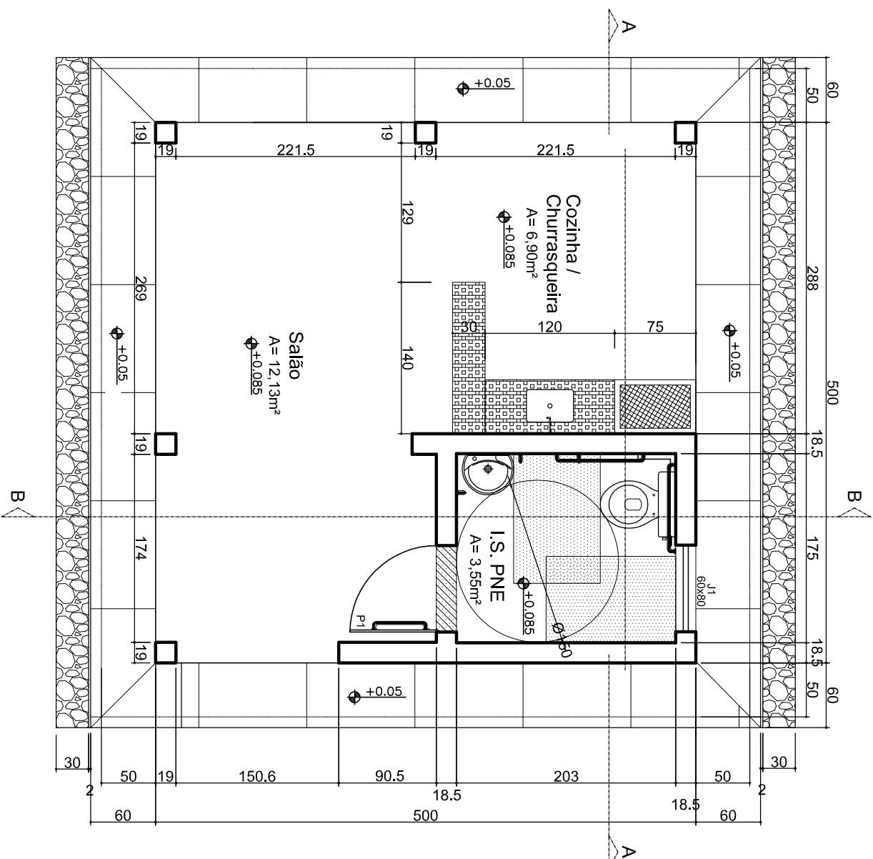
PLANTA CENTRO COMUNITÁRIO escala 1/50
