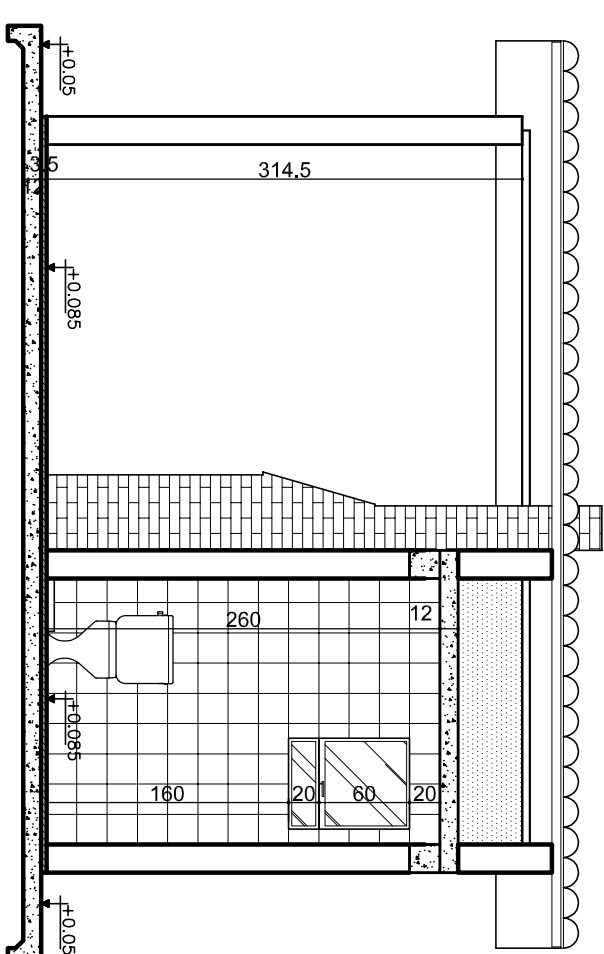
CORTE AA CENTRO COMUNITÁRIO escala 1/50
