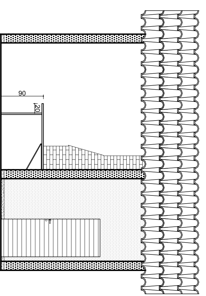
ELEVAÇÃO LATERAL escala 1/50
