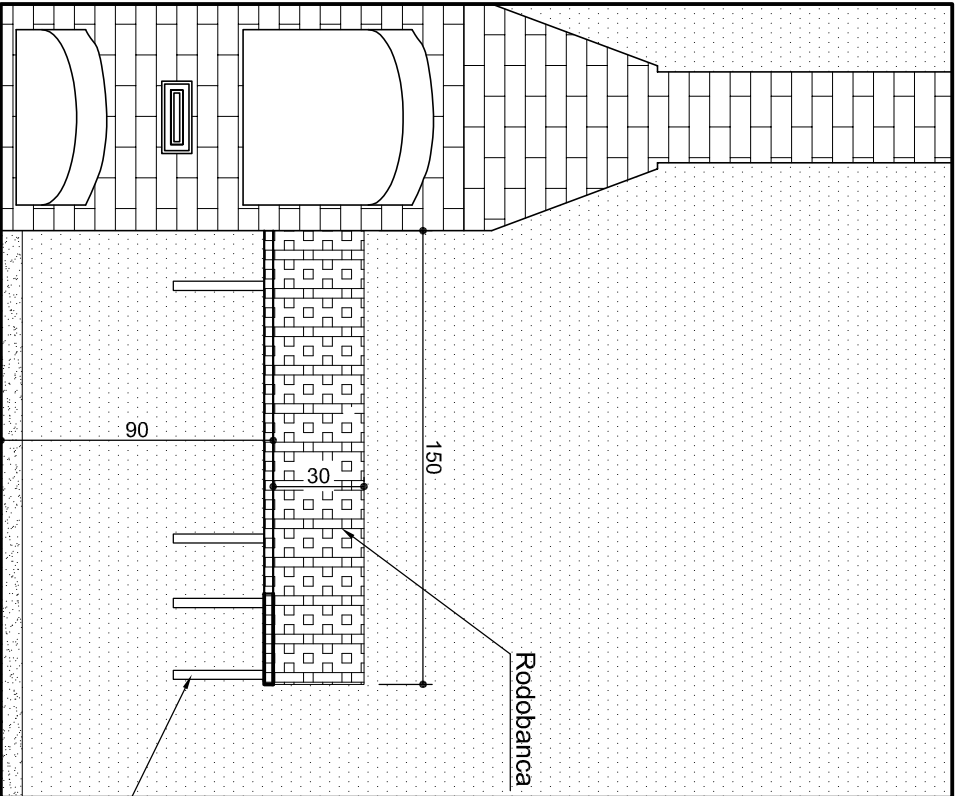
PAGINAÇÃO - VISTA 1 escala 1/25
