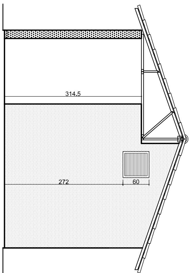
ELEVAÇÃO POSTERIOR escala 1/50
