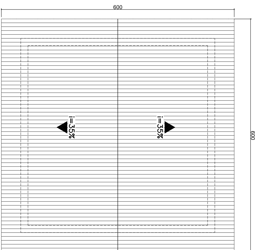
DIAGRAMA DE COBERTURA CENTRO COMUNITÁRIO escala 1/50
