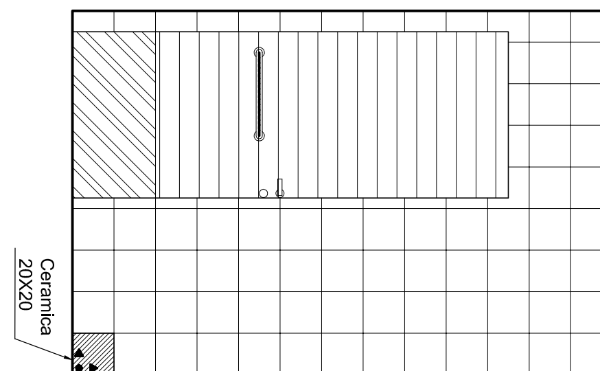
PAGINAÇÃO - VISIA 6 escala 1/25
