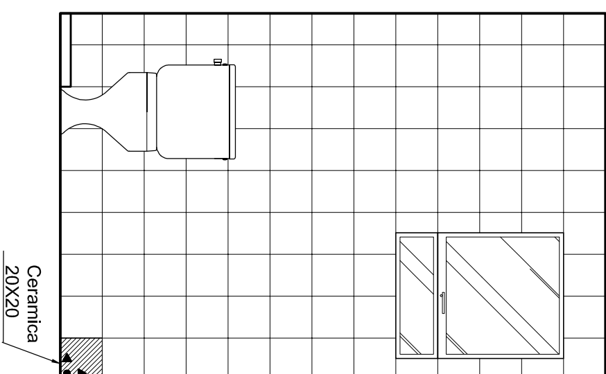
PAGINAÇÃO - VISTA 4 escala 1/25
