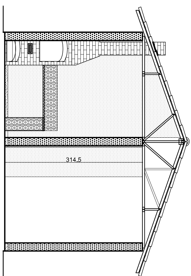
ELEVAÇÃO FRONTAL escala 1/50
