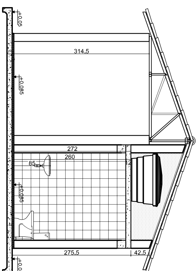
CORTE BB CENTRO COMUNITÁRIO escala 1/50
