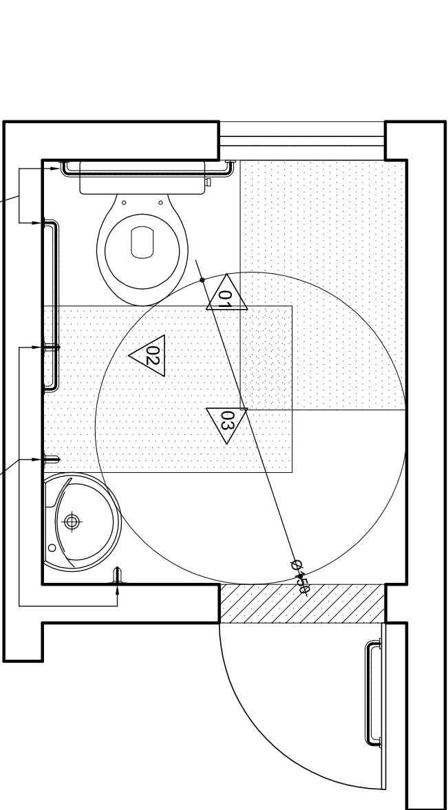
escala 1/25 PLANTA BANHEIRO COLETIVO PNE INDICATIVA DAS VISTAS
